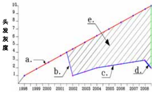
lzm 实验-基因还原曲线图
